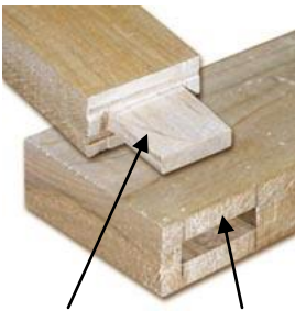
Tenon, Mortaise
